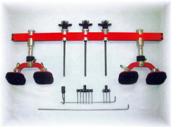
FAN Multiquick-System Art.Nr.0205
