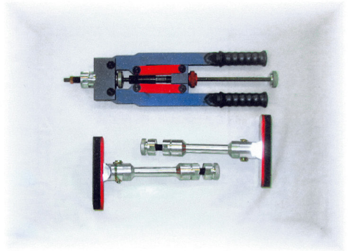
mit FAN Multiquick-System Zugzange Art.Nr. 0210
